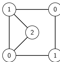
Figure 2 : Le graphe colorié avec trois « couleurs » (0, 1 et 2)
