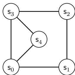
Figure 1 : Un graphe d'ordre cinq
